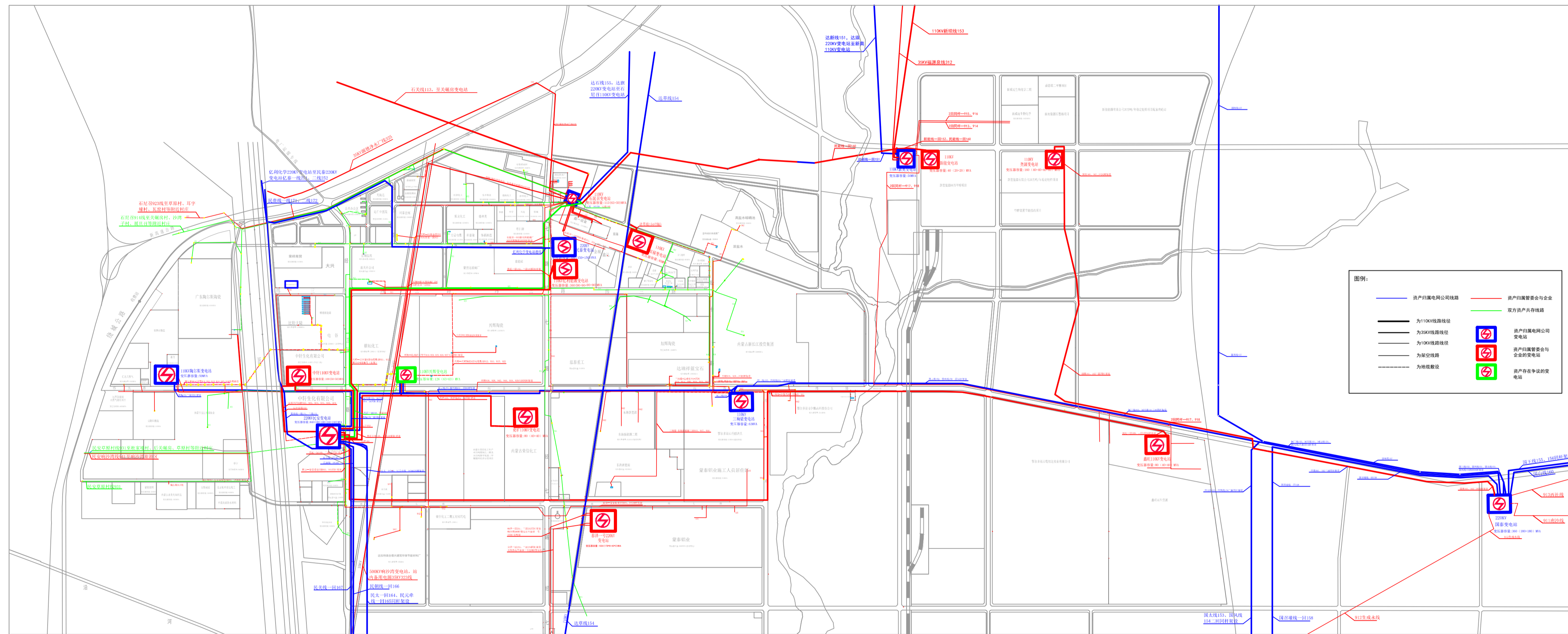
内蒙古达拉特经济开发区配电线路图
